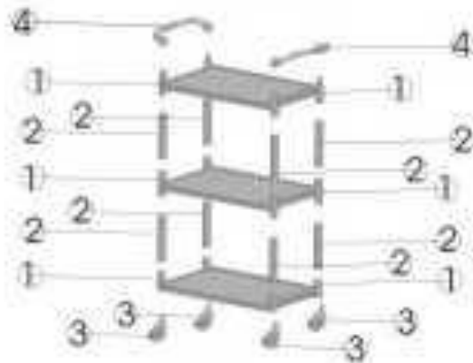
Чертеж сборки
