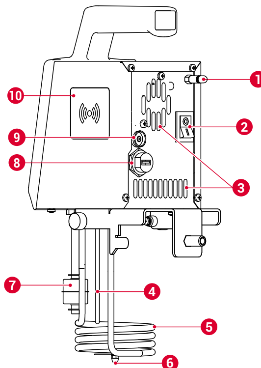
Fig. 1: SmartVide X/XL, principaux composants, partie 1
